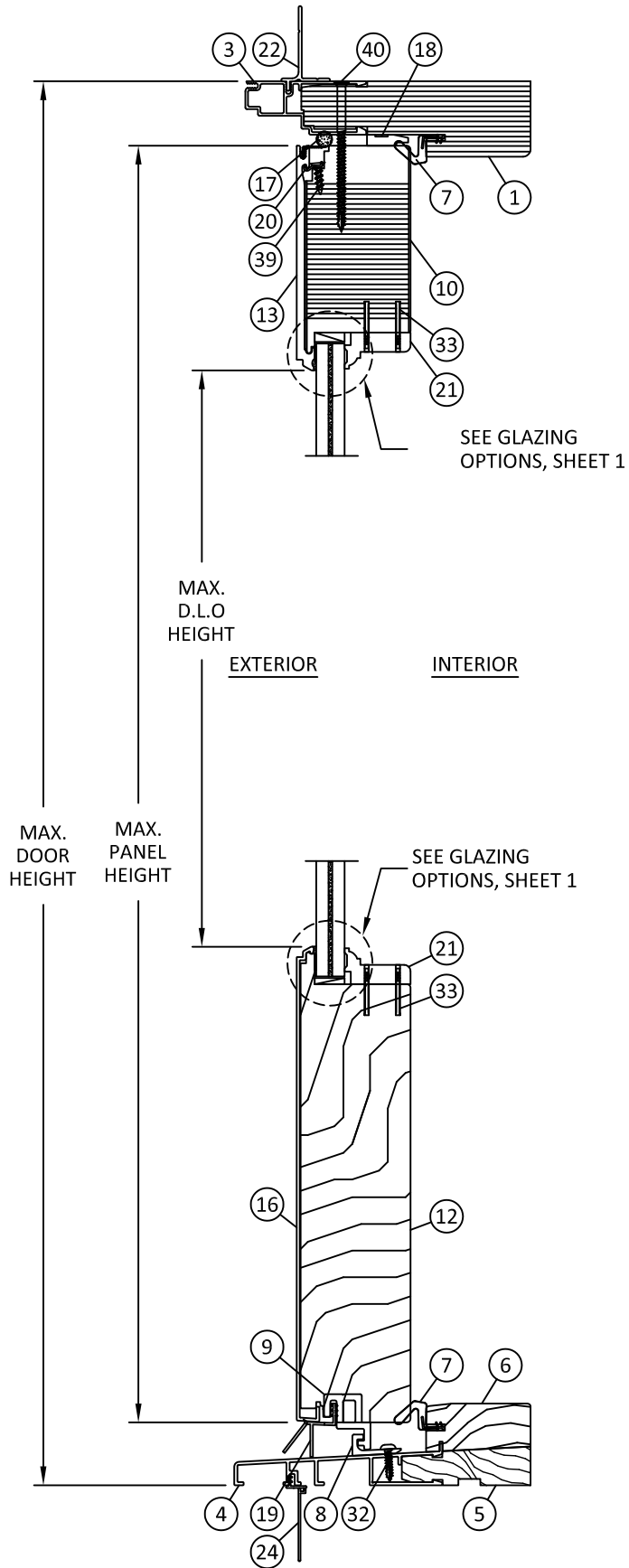
B 7 VERTICAL SECTION NAIL FIN FIXED DOOR
